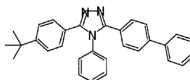
3-(4-tert-butylphenyl)-4-phenyl-5-(4-biphenyl)-1,2,4-triazole
